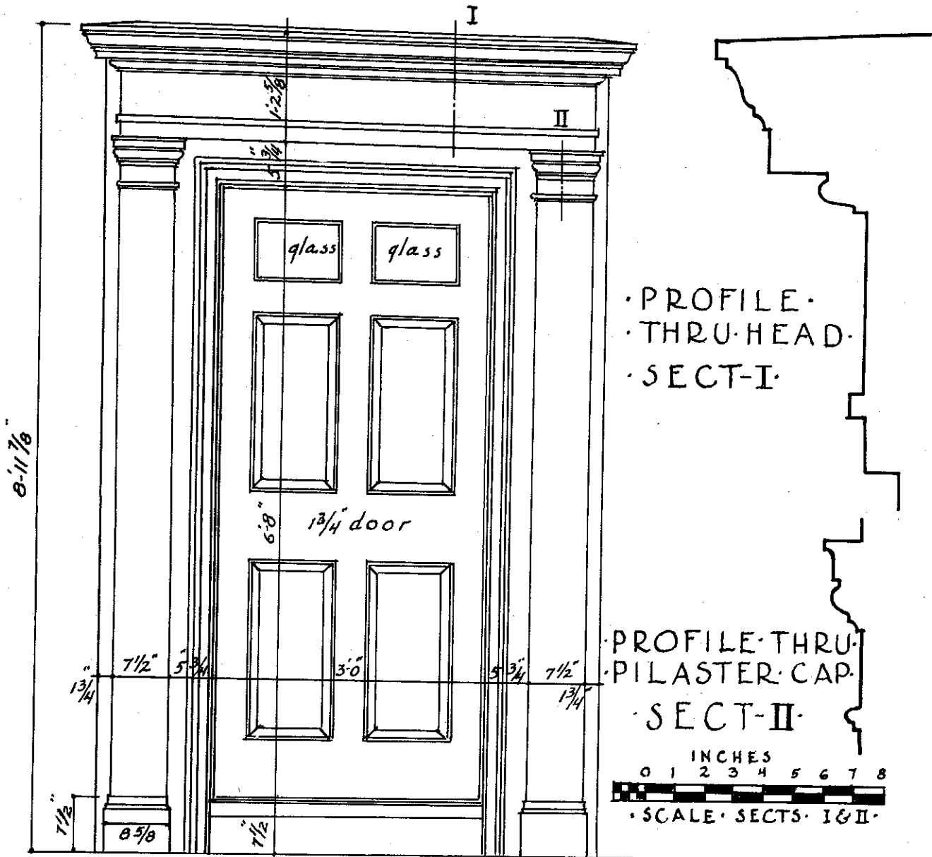
·FRONT·ELEV·
